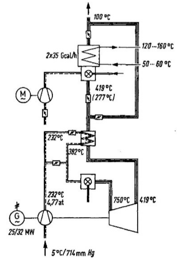
Abb. 719. Heizkraftwerk München-Sendling, Block 1 und 2
